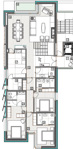
PISO 2
