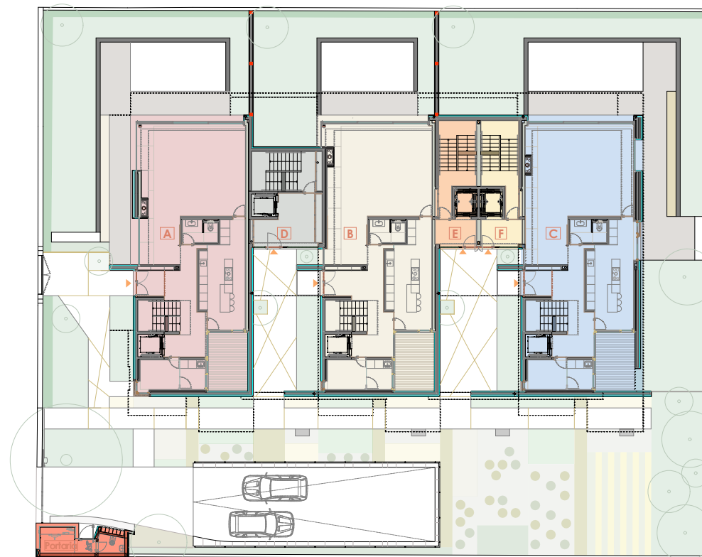
PLANTA DO PISO TÉRREO
