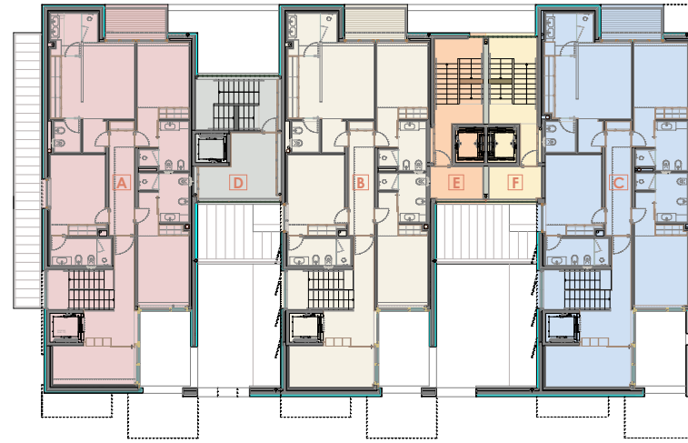
PLANTA DO 1º PISO
