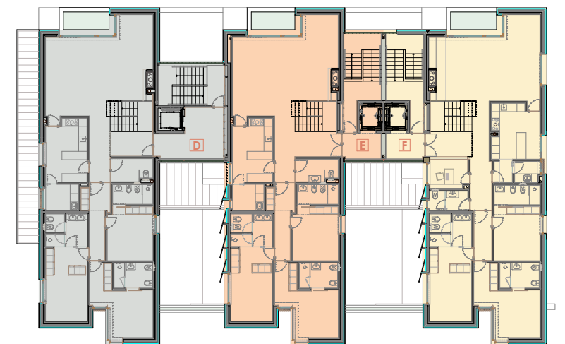
PLANTA DO PISO RECUADO
